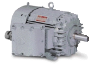
내압 방폭형 전동기
